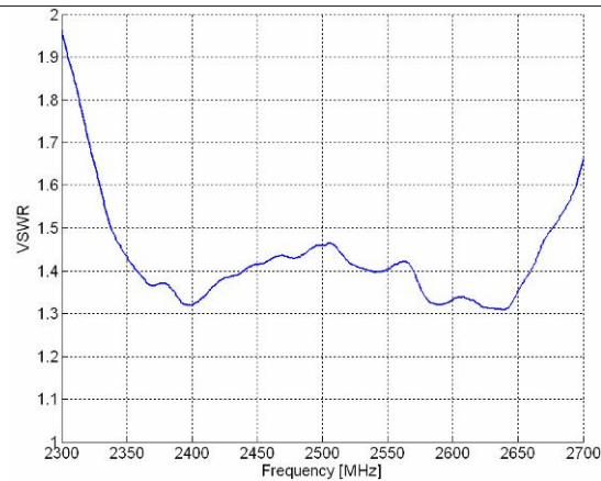
VSWR
